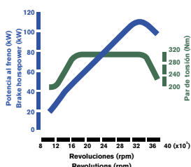
Curva de rendimiento del motor ZD30DDT (CEE) ZD30DDT Engine performance curve (EEC)
